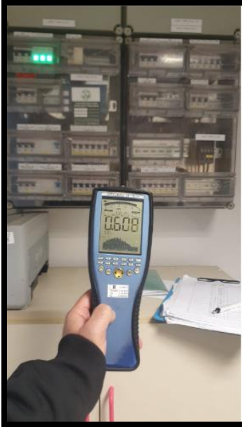
תמונה 4: הערך המתקבל בחזית לוח מקלט
